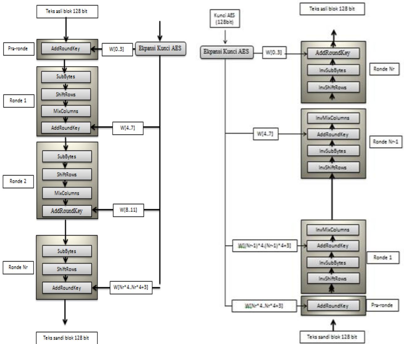
Gambar 1. Proses enkripsi dan dekripsi
