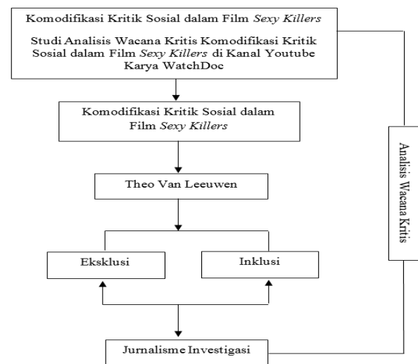
Gambar 1. Kerangka Pemikiran
